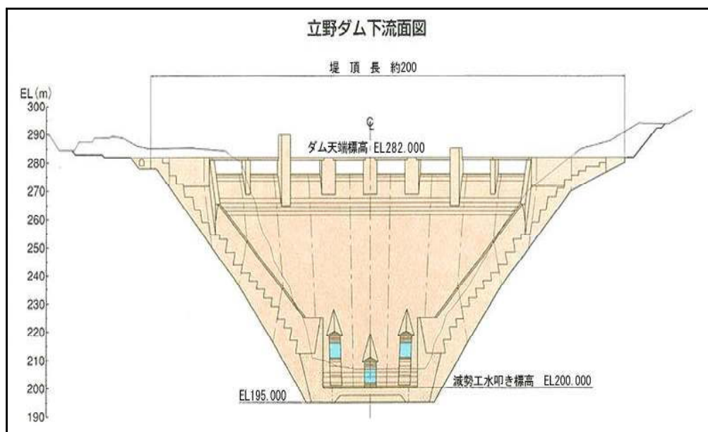
ダム上部に8つの非常放水用の穴がある立野ダム(国土交通省資料より)
